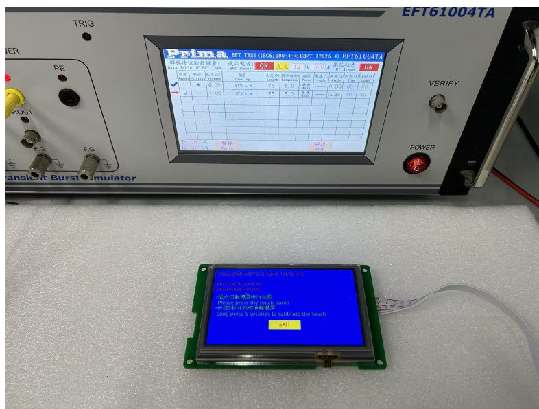
图 4-3 EFT 测试图
